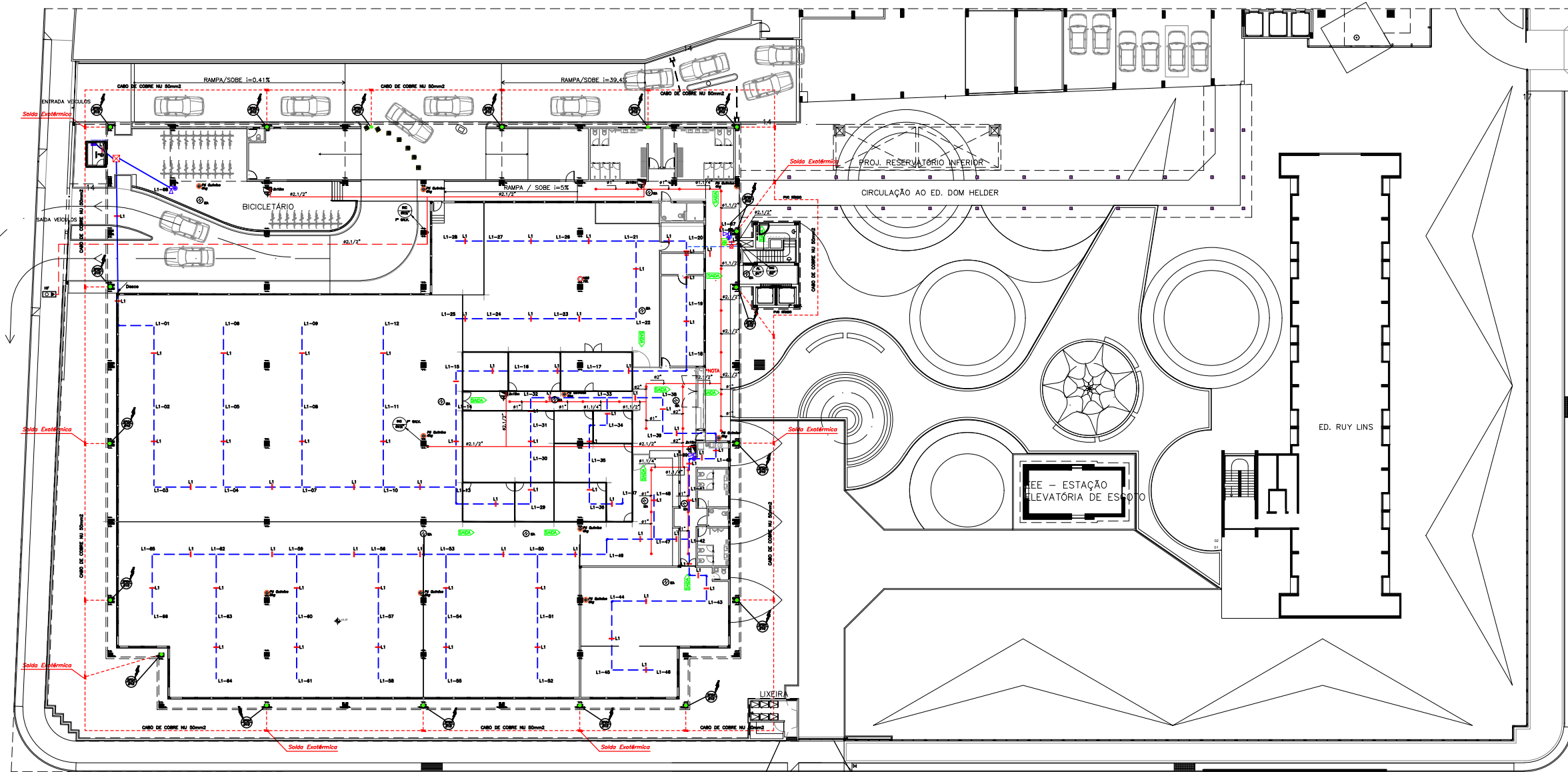
PLANTA BAIXA TÉRREO IMPLANTAÇÃO GERAL ESCALA .....1/250'
