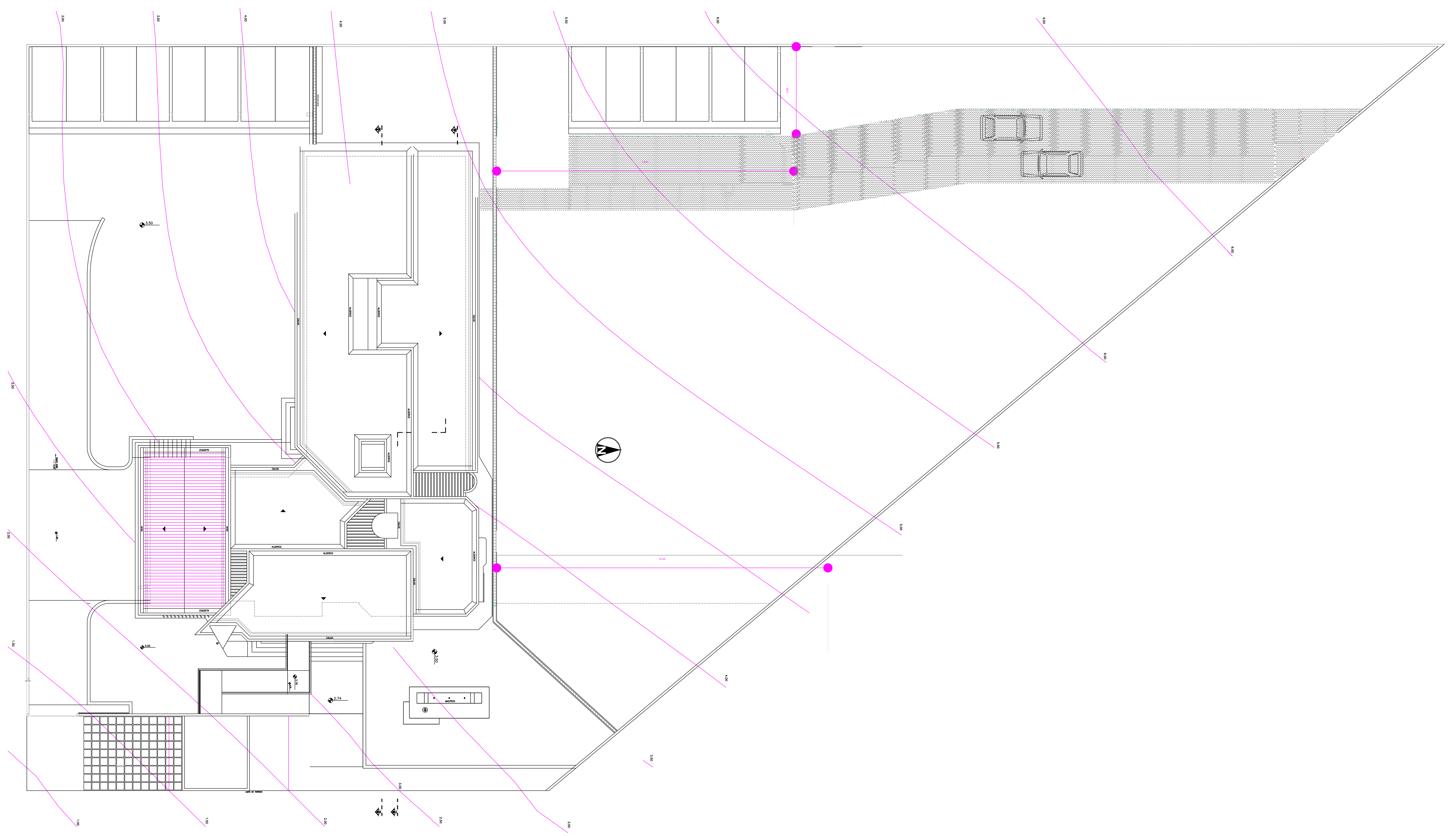
PLANTA DE COBERTA ESCALA 1:100
