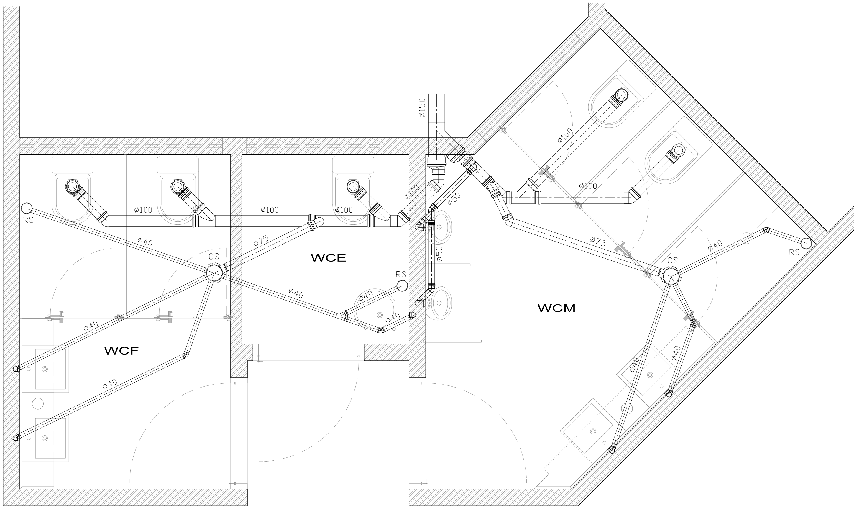
PLANTA BAIXA ESCALA ..... 1/20
