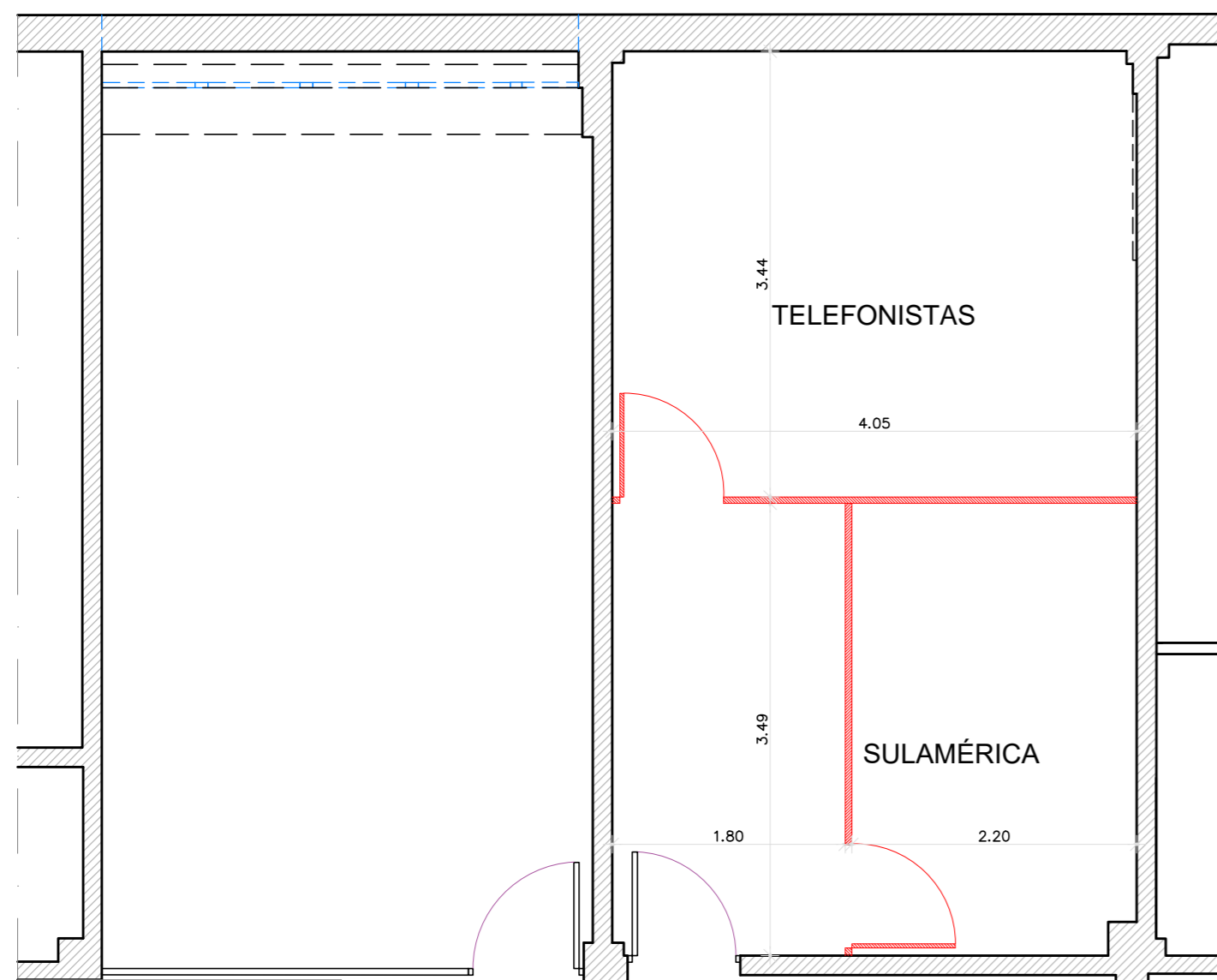
PLANTA BAIXA Construção ESCALA ..... 1/50
