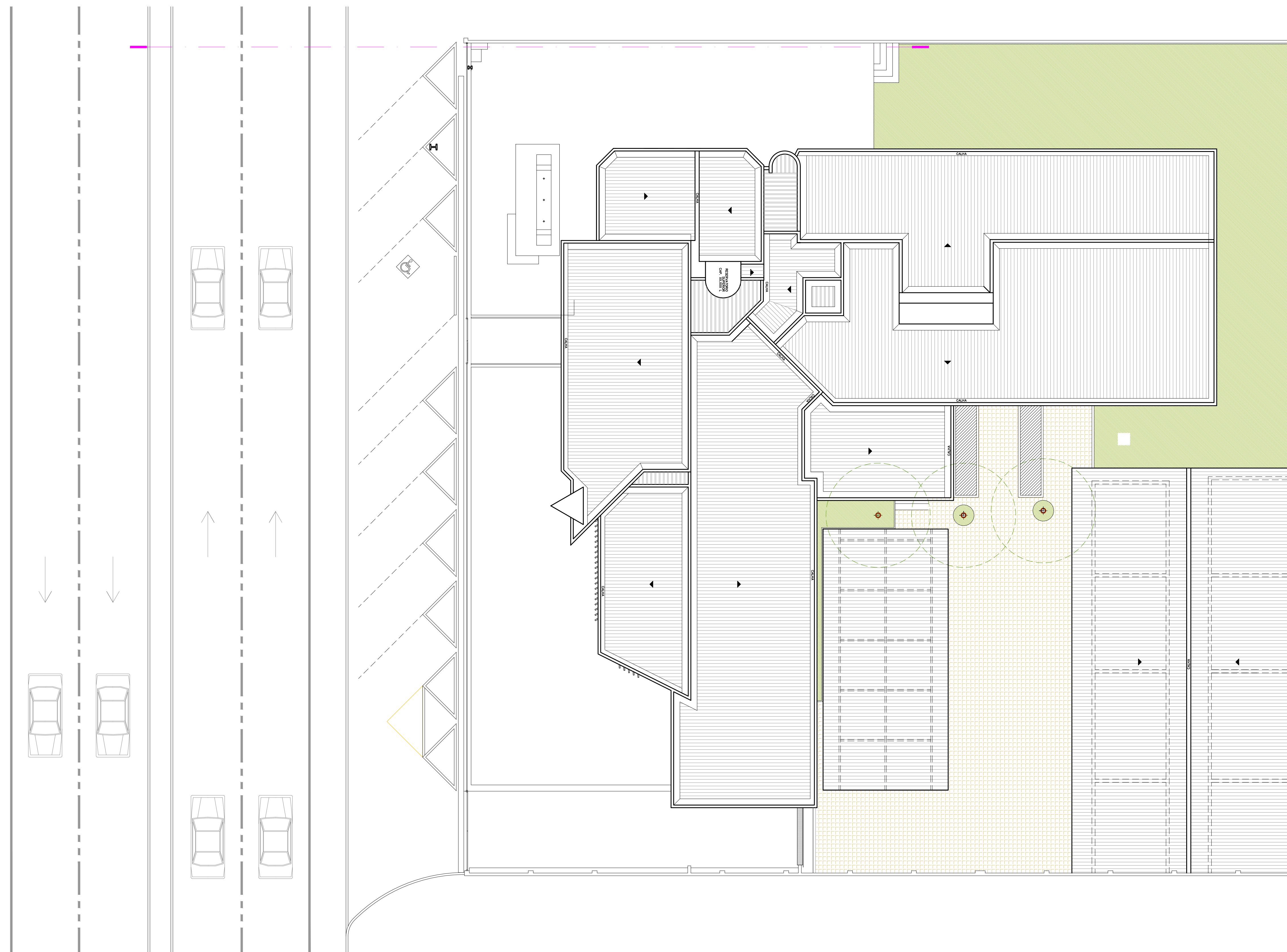
PLANTA DE COBERTA ESCALA 1/100
